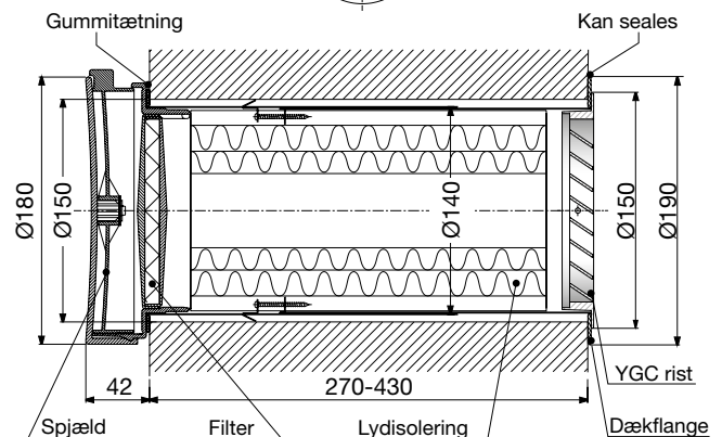
Udvendig rist type 2
