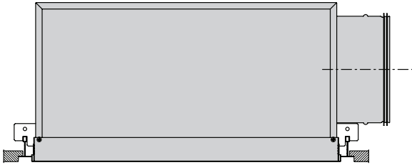
Trykfordelingsboks type H inklusive montagebeslag type PBB.
