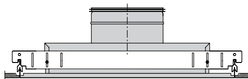
Overpart type V inklusive montagebeslag type PBB.
