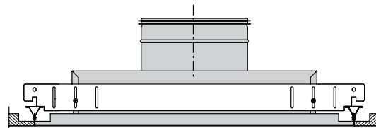
Overpart type V inklusive montagebeslag type PBB.
