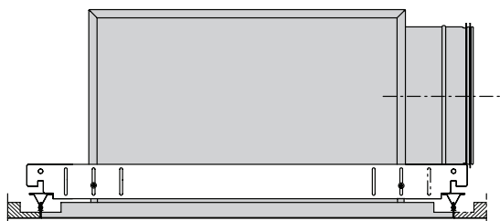
Trykfordelingsboks type H inklusive montagebeslag type PBB.
